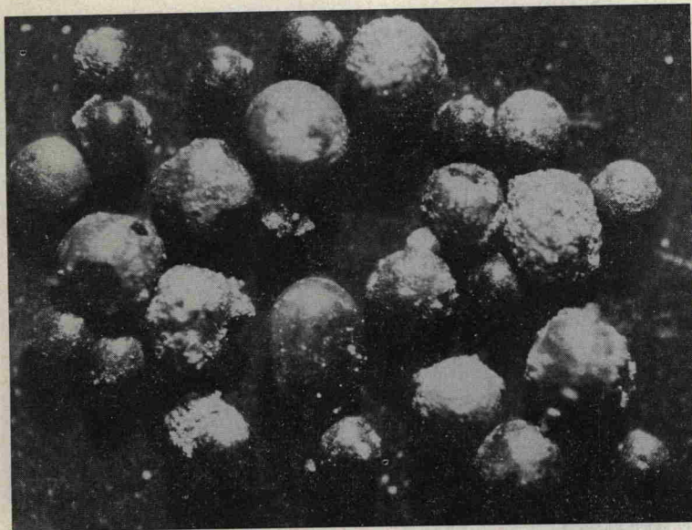
Abb. 10. Glaskugeln aus dem Mondboden von der Landestelle von Apollo 11 im Meer der Ruhe (Mare Tranquillitatis), Durchmesser der Kugeln: 0,25 bis 0,5 mm.
